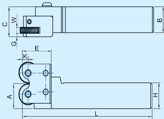
右手系 Right-hand shown
