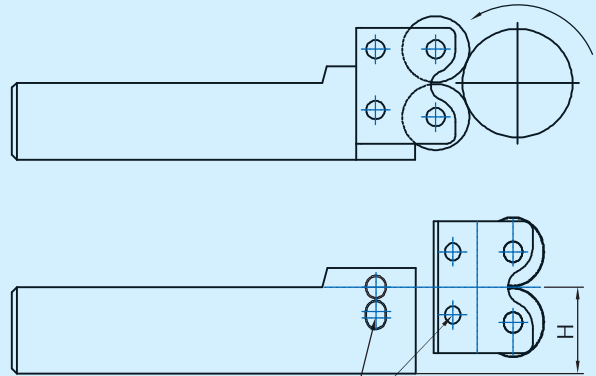
使用雙輪刀片螺絲鎖緊的位置 Locking Screw Position For Two Knurling Rolls
