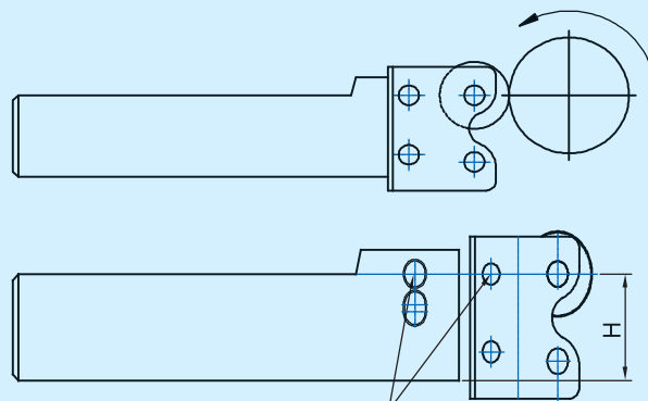
使用單輪刀片螺絲鎖緊的位置 Locking Screw Position For Single Knurling Roll
