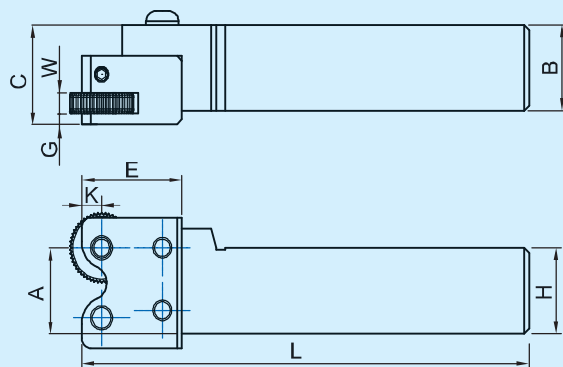
右手系 Right-hand shown
